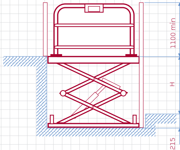
Wall shaft/Mauerschacht
